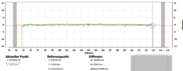
Profil vor Microfinish
