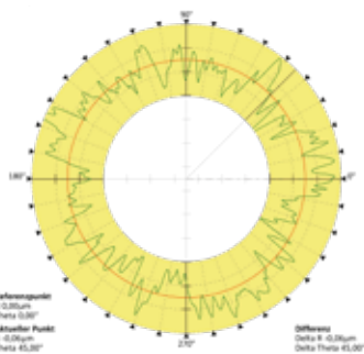
Rundheit vor Microfinish
