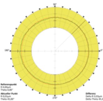
Rundheit nach Microfinish
