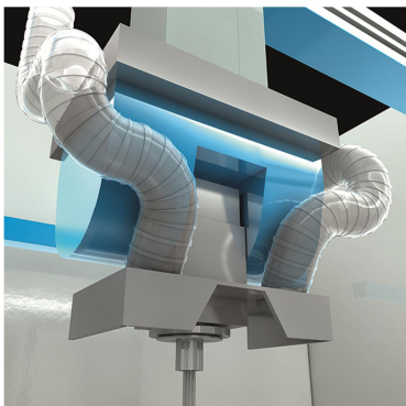
Bild 2: Die beim Fräsen frei werdenden feinen Fasern müssen zuverlässig abgesaugt werden.
