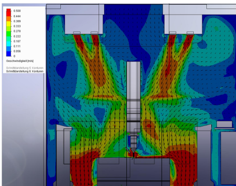
Bild 3: Die Erfassung der Stäube war eine Herausforderung - die Strömungssimulation half, eine maßgeschneiderte Lösung zu finden.
